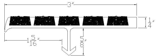
Type 231BF
